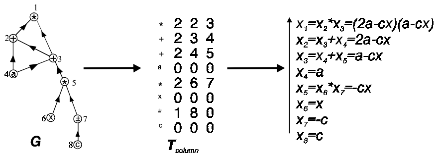
Obrázok 5.25. Ilustračný príklad výpočtu funkčných hodnôt syntaktického grafu G z obr. 5.22, ktorého jednotlivé vrcholy sú teraz ohodnotené algebraickými operáciami. Stĺpcová tabuľka T v tomto prípade je rozšírená o nový 0-tý stĺpec, ktorý špecifikuje funkcie priradené jednotlivým vrcholom. Výsledné ohodnotenie syntaktického grafu je funkčná hodnota výstupného vrcholu (2a-cx)(a-cx) .
