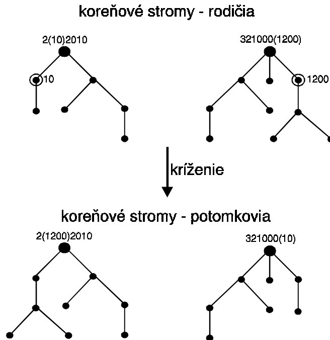
Obrázok 5.7. Ilustratívny príklad operácie kríženia dvoch rodičovských koreňových stromov, ktoré sú modifikované na dva nové koreňové stromy - potomkov. Zakrúžkované vrcholy označujú náhodne generované body kríženia. Operácia kríženia spočíva v tom, že podstromy sa medzi koreňovými stromami vymenia.
