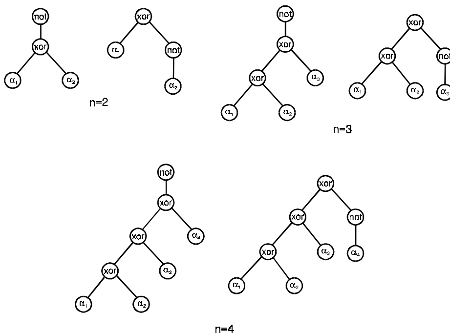
Obrázok 5.29. Syntaktické stromy pre Boolovskú funkciu parity vyjadrenú výrazmi (5.53a-b).
