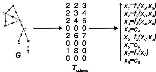
Obrázok 5.24. Ilustračný príklad výpočtu funkčných hodnôt syntaktického grafu G určeného pomocou stĺpcovej tabuľky T_{column} . Postupujúc zdola-hore cez všetky riadky tabuľky, funkčné hodnoty sú rekurentne počítané pomocou predchádzajúcich funkčných hodnôt.
