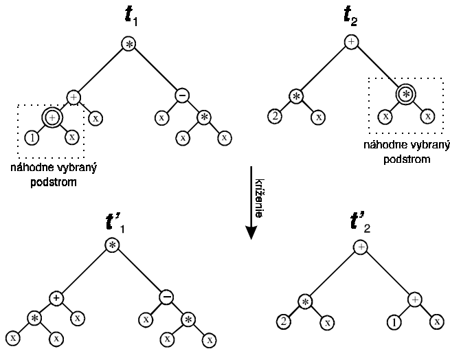
Obrazok 5.15. Ilustračný príklad kríženia dvoch syntaktických stromov. V prvej etape v každom strome sa náhodne vyberie podstrom, v druhej etape sa tieto podstromy vzájomne zamenia. Formálne môžeme povedať, že operáciou kríženia sa dve funkcie t_1(x) a t_2(x) pretransformovali na nové funkcie t_1'(x) a t_2'(x) .
