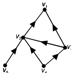
Obrázok 5.21. Orientovaný graf obsahujúci päť vrcholov a šesť orientovaných hrán. Množina vrcholov V obsahuje päť vrcholov, V = \{v_1, v_2, v_3, v_4, v_5\} , množina hrán obsahuje šesť orientovaných hrán, E = \{e_1, e_2, e_3, e_4, e_5, e_6\} . Orientovaná e \in E je určená pomocou usporiadanej dvojice dvoch vrcholov v, v' \in E , e = (v, v') . Hovoríme, že orientovaná hrana e začína v o vrchole v (hrana e vzhádza z vrcholu v ) a končí vo vrchole v' (hrana e vchádza do vrcholu v' ). Graf je acyklický, neobsahuje cyklickú cestu, ktorá by sa skladala z postupnosti rovnako orientovaných hrán.
