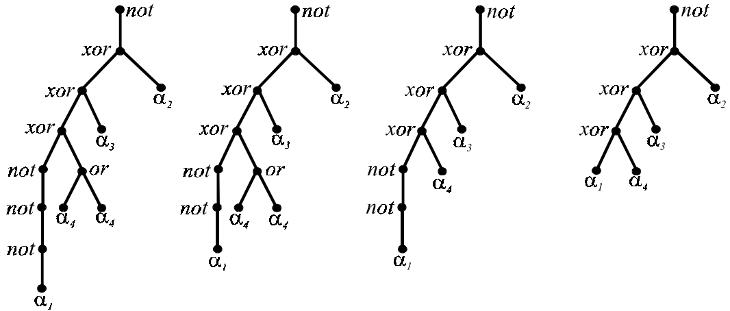
Obrázok 5.31. Znáznornenie syntaktických stromov produkovaných genetickým programovaním pre symbolickú regresiu parity binárnych vektorov dimenzie n=4 . Všetky tieto stromy majú nulovú hodnotu účelovej funkcie (5.26), penalizačný člen z príkladu (5.7) zvyhodňuje tie stromy, ktoré majú menší počet vrcholov. Posledný strom je totožný so stromom na obr. (5.29), takže môžeme konštatovať, že v tomto jednoducho prípade symbolickej regresie, genetické programovanie poskytuje optimálny výsledok.
