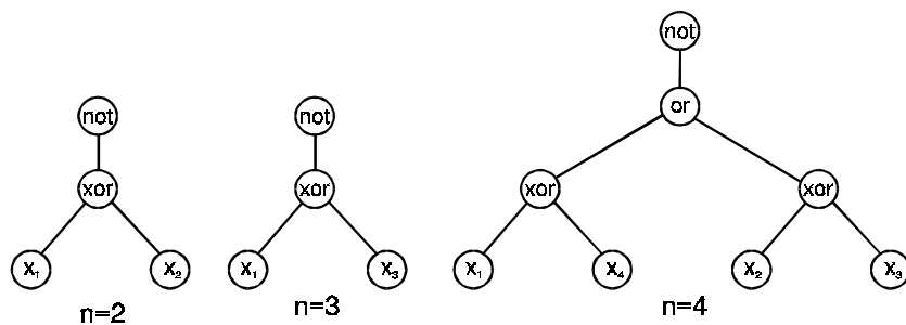
Obrázok 5.30. Syntaktické stromy Boolovských výrazov vyjadrujúcej symetriu binárnych reťazcov podľa výrazov (5.55).
