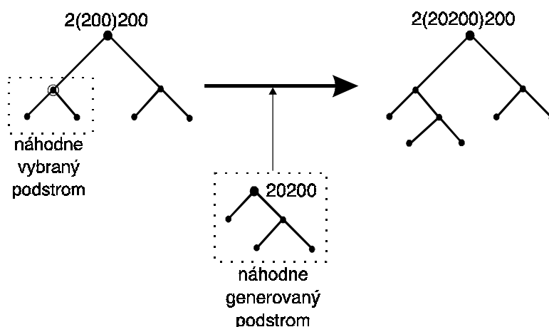
Obrázok 5.6. Ilustratívny príklad mutácie koreňového stromu. V prvom kroku je náhodne vybraný nekoreňový vrchol, ktorý je zakružkovaný na ľavom koreňovom strome. Príslušný koreňový podstrom je nahradený iným náhodne generovaným koreňovým podstromom. Počiatočný a konečný kód príslušných koreňových stromov sú uvedené pri koreňových vrcholoch.
