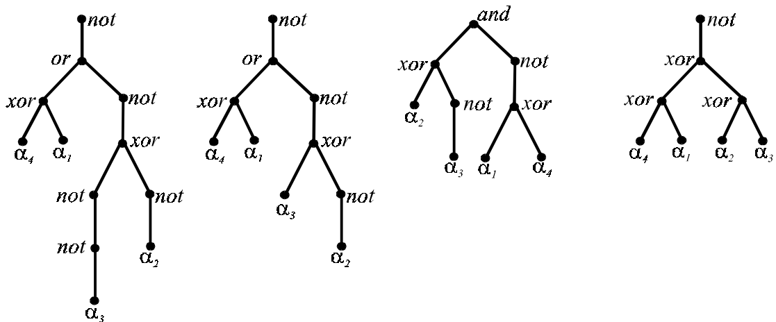
Obrázok 5.32. Syntaktické stromy pre parity binárnych vektorov dimenzie n=4 . Posledný strom je totožný so stromom na obr. 5.30. v tomto špeciálnom prípade, genetické programovanie opäť poskytuje správny výsledok.
