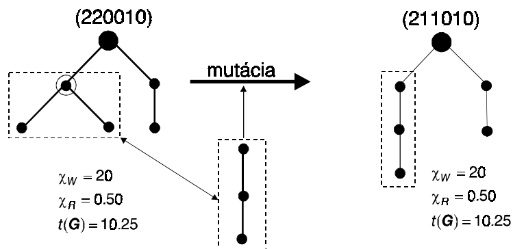
Obrázok 5.19. Ilustračný príklad mutácie koreňového stromu, podstrom susedný s náhodne vybraným vrcholom (zakrúžkovaný) sa vymení za náhodne vygenerovaným podstromom. Hodnoty topologických indexov a príslušná vlastnosť sú uvedené pod grafmi.
