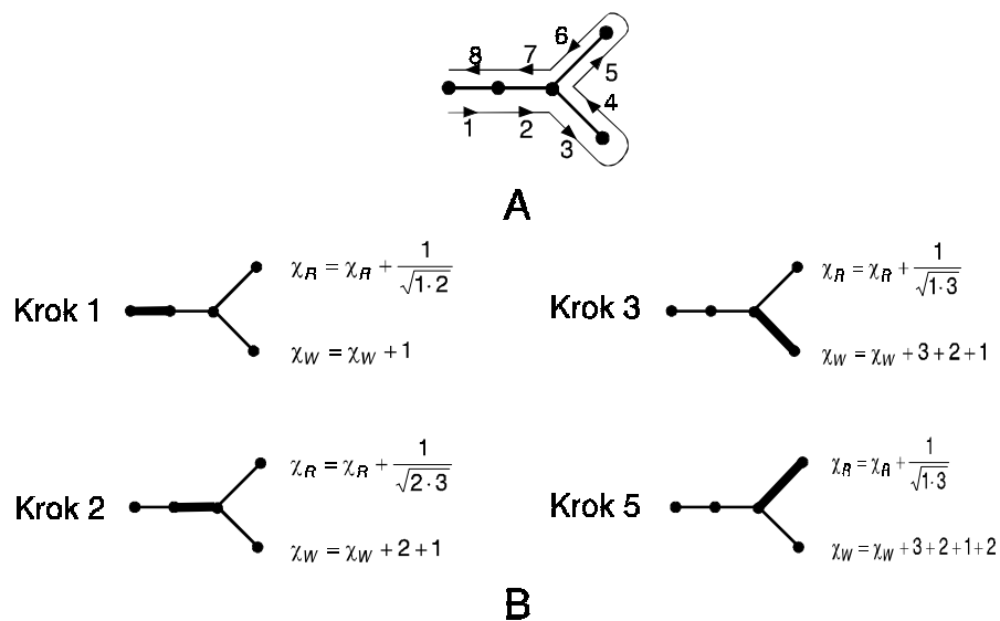
Obrázok 5.18. V priebehu analýzy koreňového stromu (diagram A) sú identifikované hrany grafu. V priebehu každého kroku tejto identifikácie vykoná sa čiastočný výpočet Randičovho a Wienerovho indexu (diagram B).
