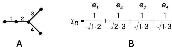
Obrázok 5.17. Výpočet Randičovho topologického indexu pre strom znázornený diagramom A, kde jednotlivé hrany stromu sú indexované. V diagrame B je priradený ku každej hrane odpovedajúci výraz 1/\sqrt{\text{val}(v) \cdot \text{val}(v')} .
