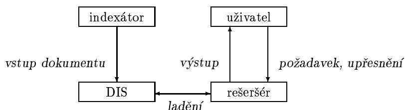
Obrázek 4: Schéma dokumentografického informačního systému
